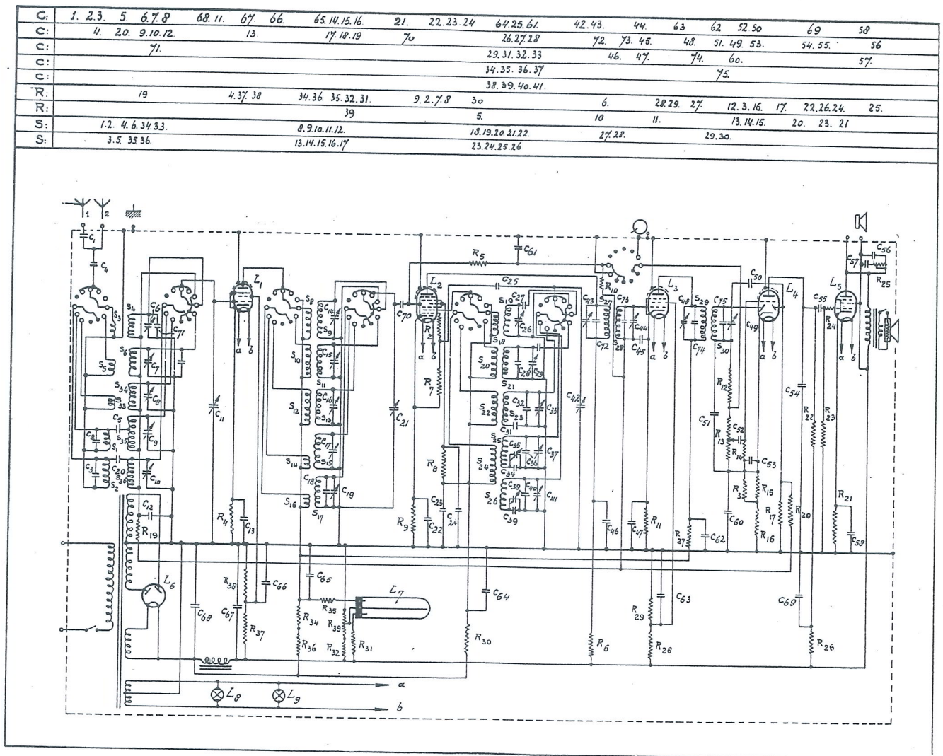
Afb. 2 Schema van de Erres K Y 149.
